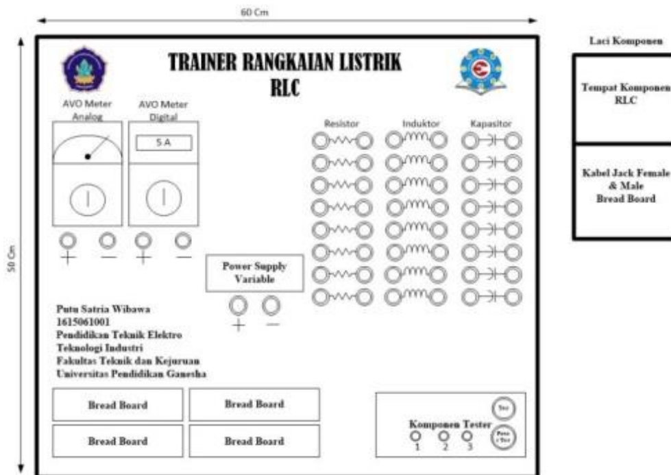
Gambar 1. Layout Desain Media Pembelajaran Rangkaian Listrik RLC
