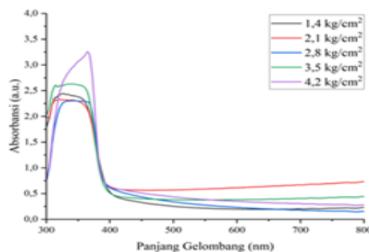
Gambar 2. Grafik Absorbansi dari Hasil Karakterisasi UV-Vis
