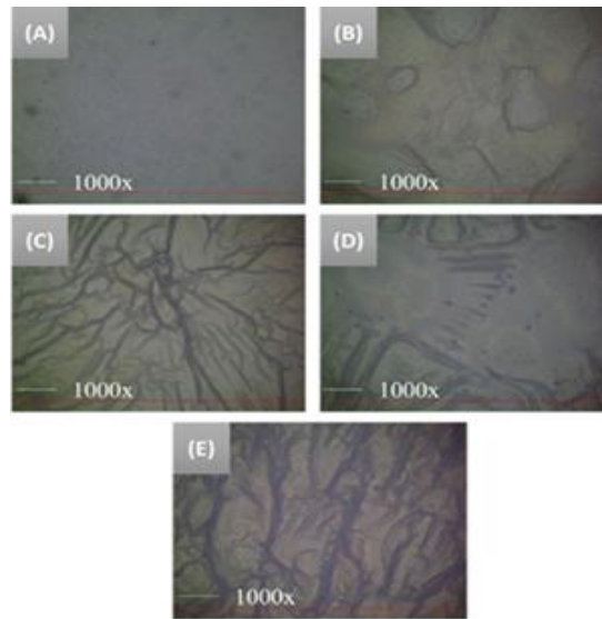
Gambar 1. Hasil Pencitraan Mikroskop CCD pada Sampel Variasi Tekanan a) 1,4 kg/cm 2 , b) 2,1 kg/cm 2 , c) 2,8 kg/cm 2 , d) 3,5 kg/cm 2 , dan e) 4,2 kg/cm 2
